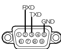
D-Sub9ピン(オス)
