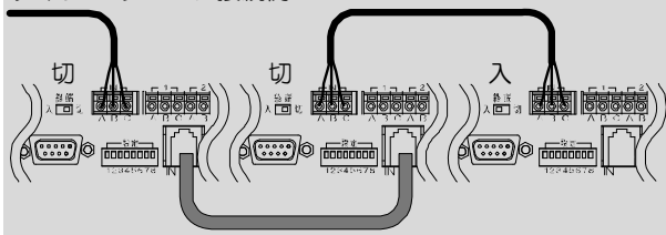
デージー チェーン接続例
