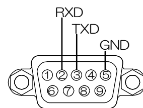
D-sub9 ピン(オス)
