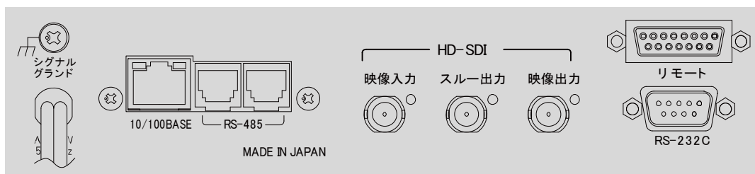
背面拡大図
