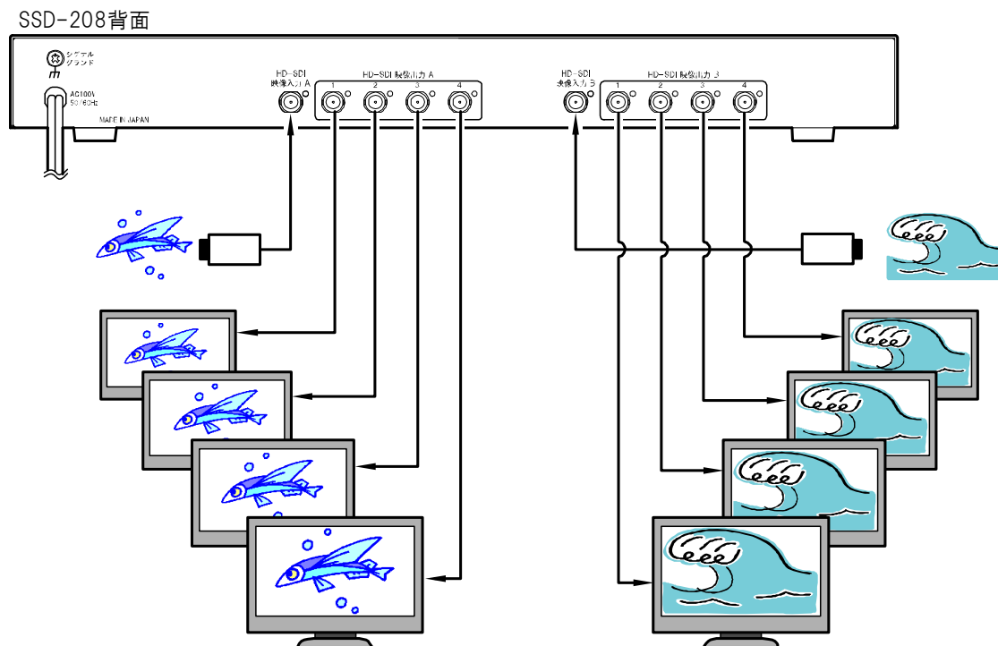
2 入力×4 分配の接続例
