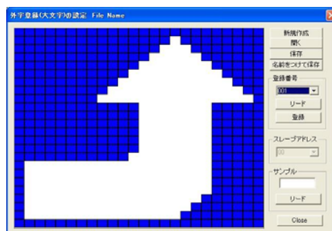
外字編集例
