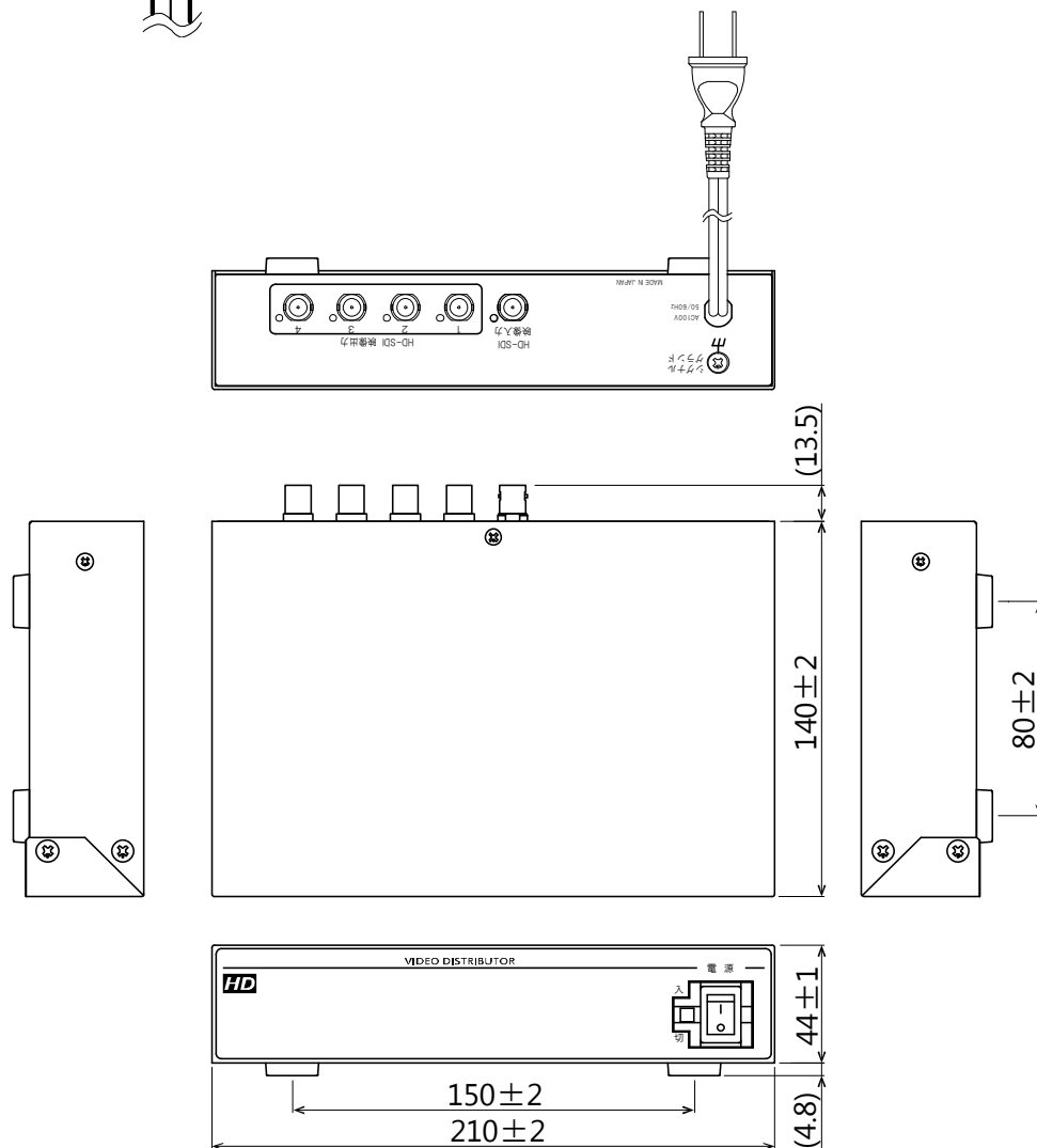
外観寸法図
