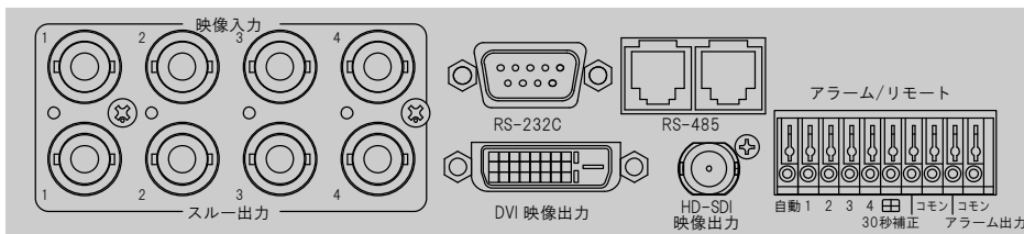
背面拡大図
